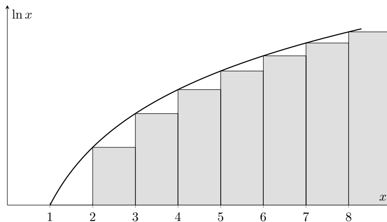
Figura 26: Interpretação do somatório como uma soma de retângulos de base 1.
