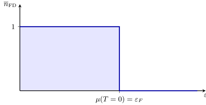
Figura 22: Distribuição de Fermi–Dirac a T = 0 . Neste contexto, o potencial químico também é chamado energia de Fermi, \varepsilon_F .
